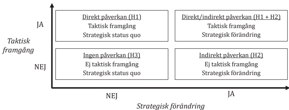
Figur 6: Hypotesernas utfallsrum.
